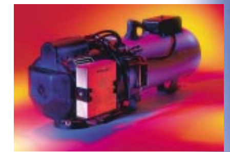
DBW 2010 : robuste et fiable, mis à l'épreuve depuis de nombreuses années. Le système de chauffage à eau avec une puissance calorifique élevée de 11,6 kW même dans des conditions extrêmes.
